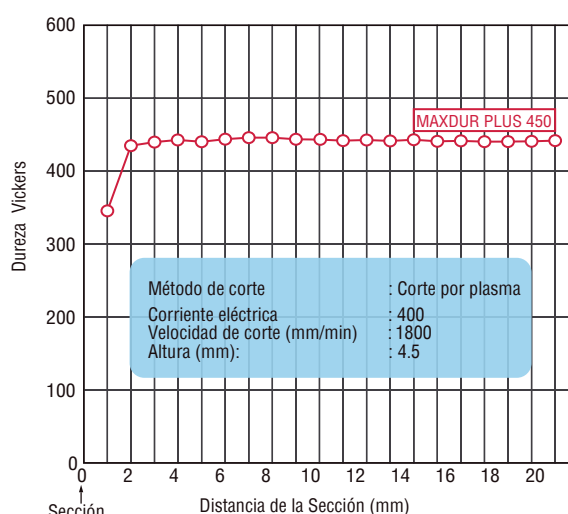
Distribución de dureza para corte por plasma
